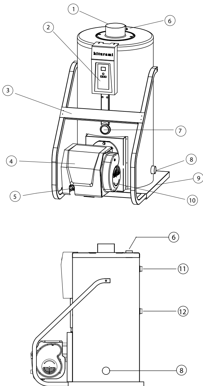
Рисунок 1. Устройство и назначение основных частей для котлов KSG 50/70
