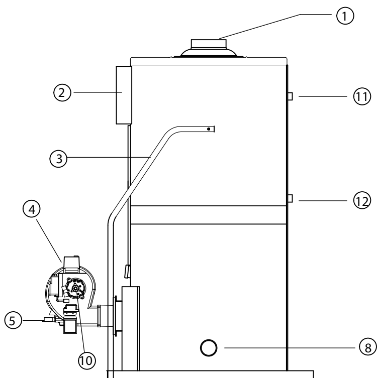
Рисунок 2. Устройство и назначение основных частей для котлов KSG-200
