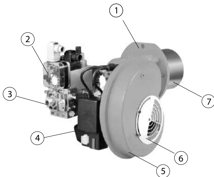
Рисунок 4. Устройство и назначение основных частей для газовой горелки TGB
