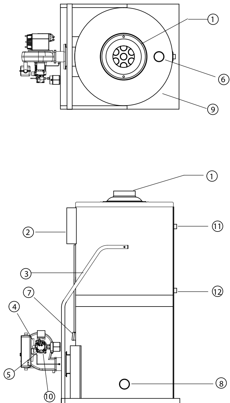
Рисунок 2. Устройство и назначение основных частей для котлов KSO-200
