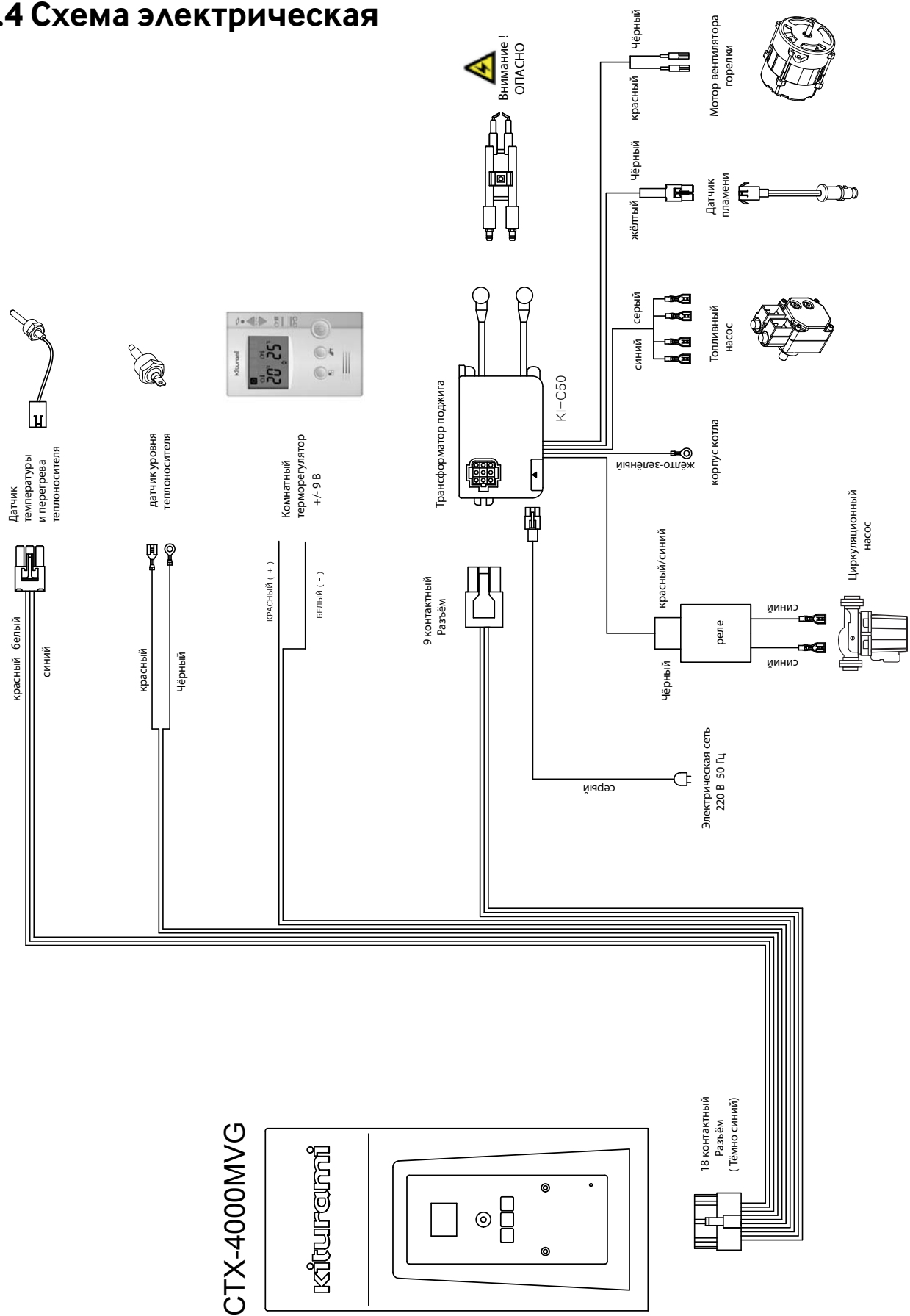
Рисунок 8. Схема электрическая для котлов KSO -50/70/100/150
