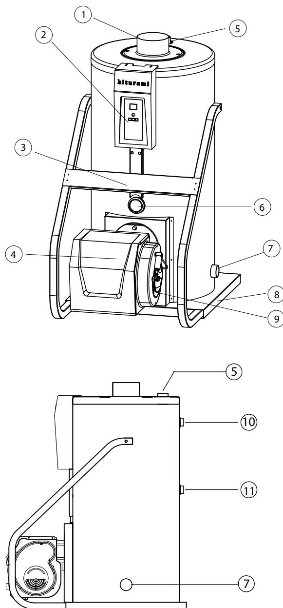
Рисунок 1. Устройство и назначение основных частей для котлов KSO- 50/70
